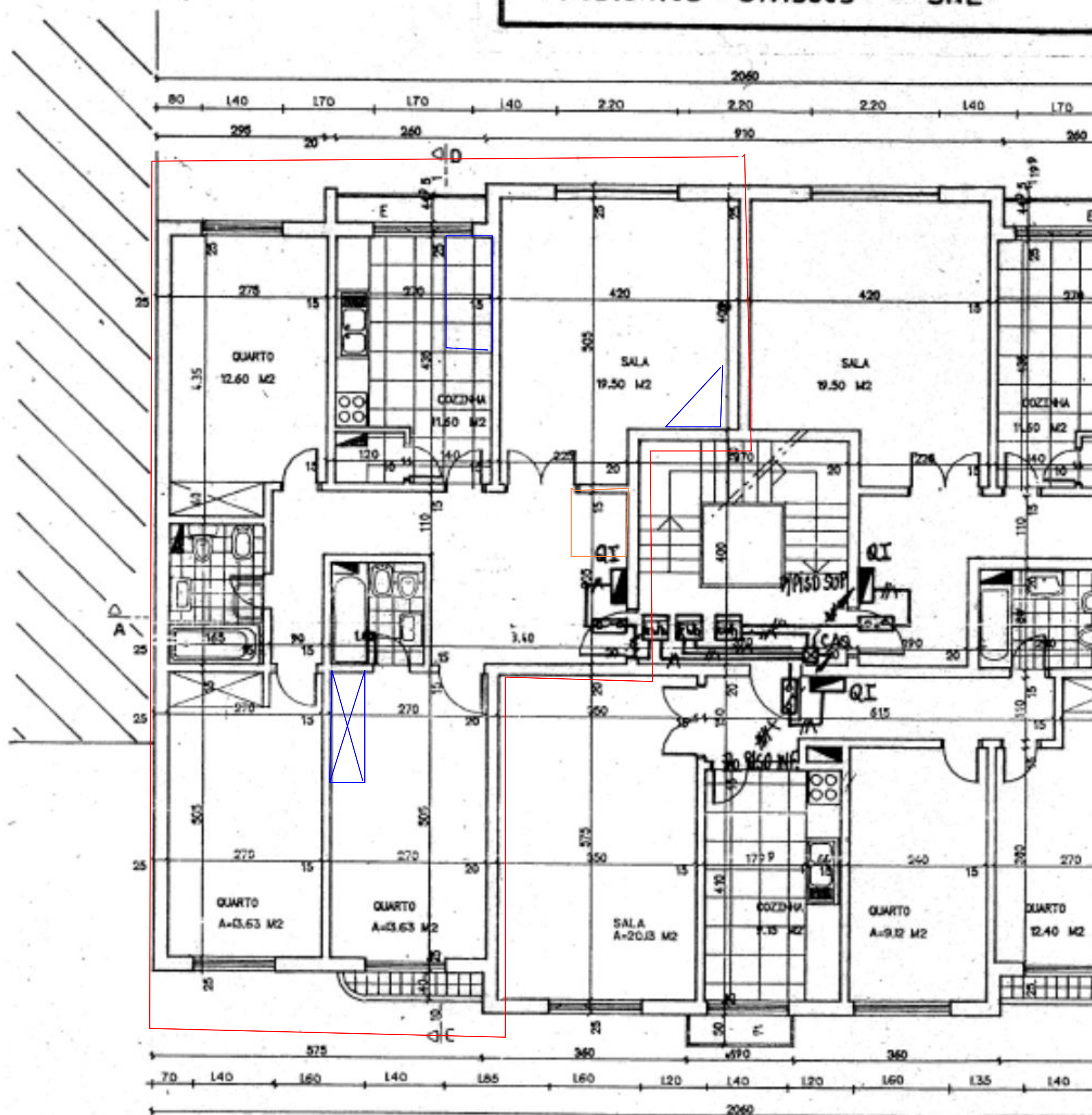
PLANTA DO ANDAR TIPO
