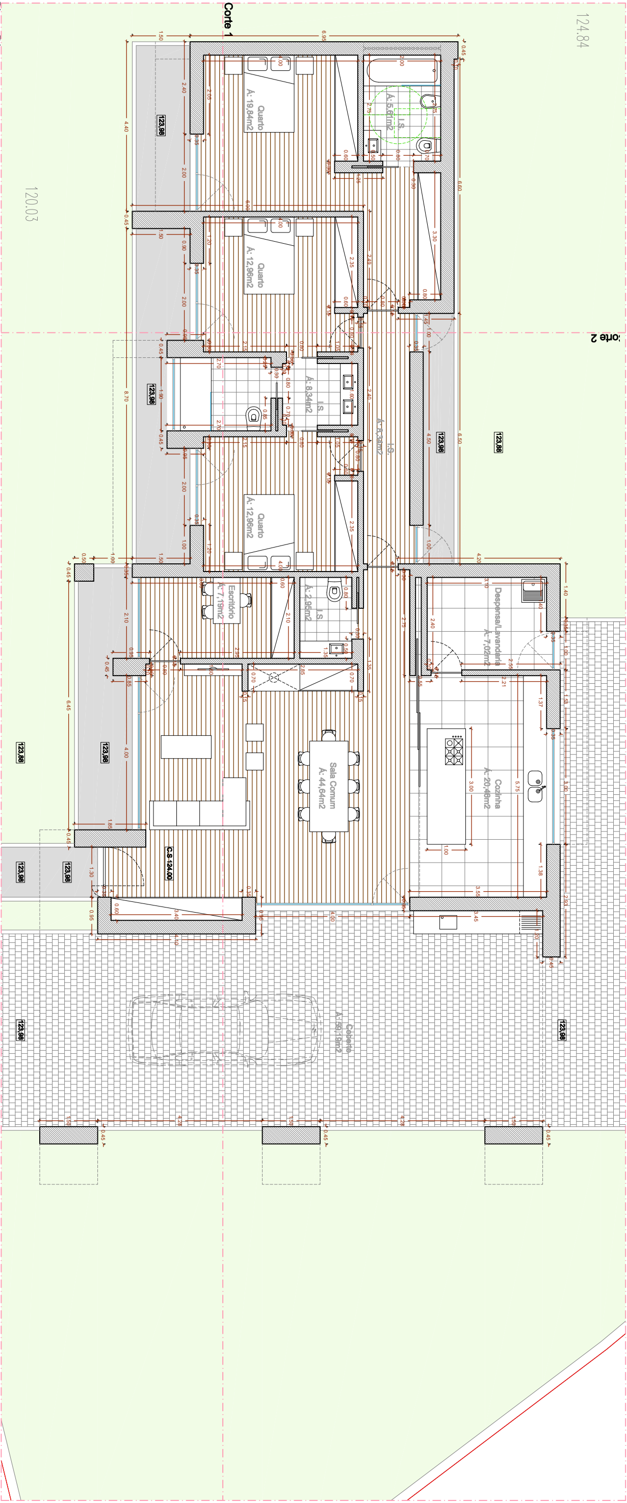
Planta R/c
