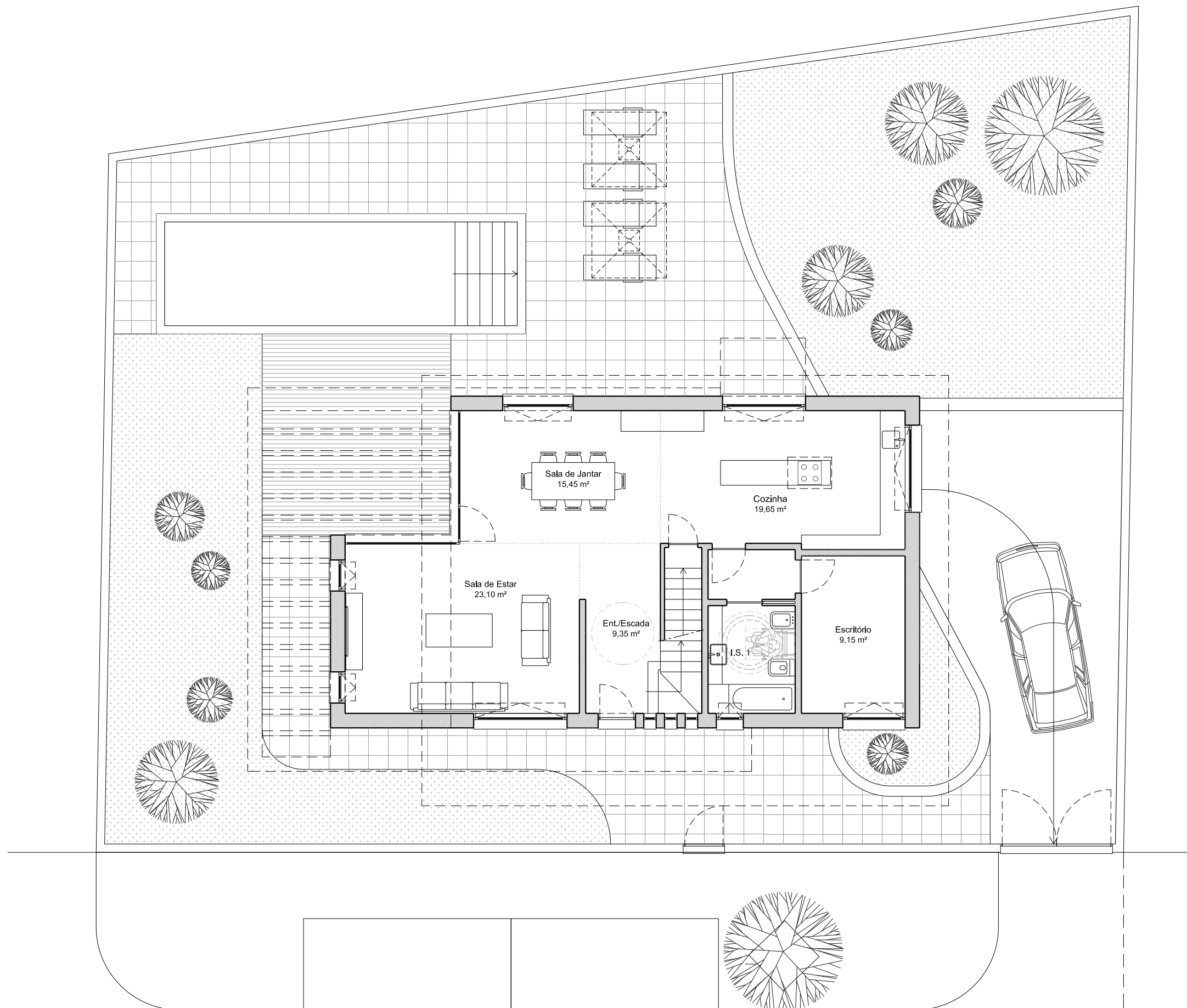
Planta do Piso 0 (Rés-do-Chão) A.B.C.: 103.90 m²
