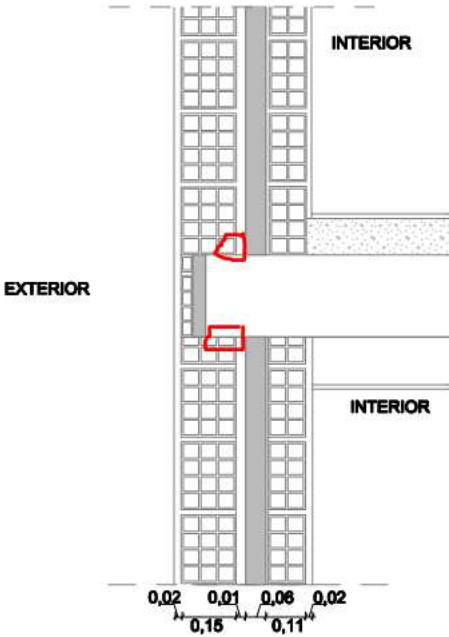
LIGAÇÃO DA FACHADA COM PAVIMENTOS I
