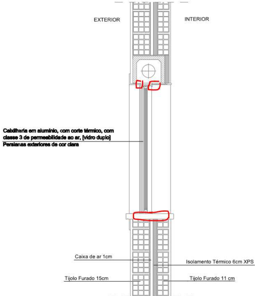
LIGAÇÃO DA FACHADA COM PADIEIRA, OMBREIRA E PEITORIL
