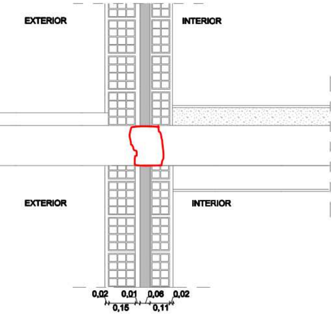
LIGAÇÃO DA FACHADA COM VARANDA
