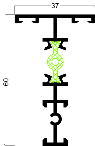
ARi-40 Divisor de vidro
