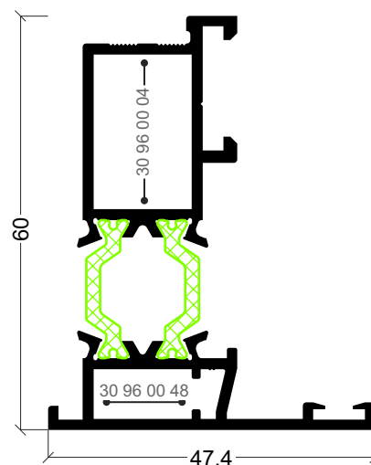
ARi-73 Inversor de sentido de abertura
