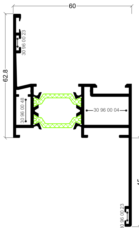
ARi-42 Aro fixo com remate folha oculta
