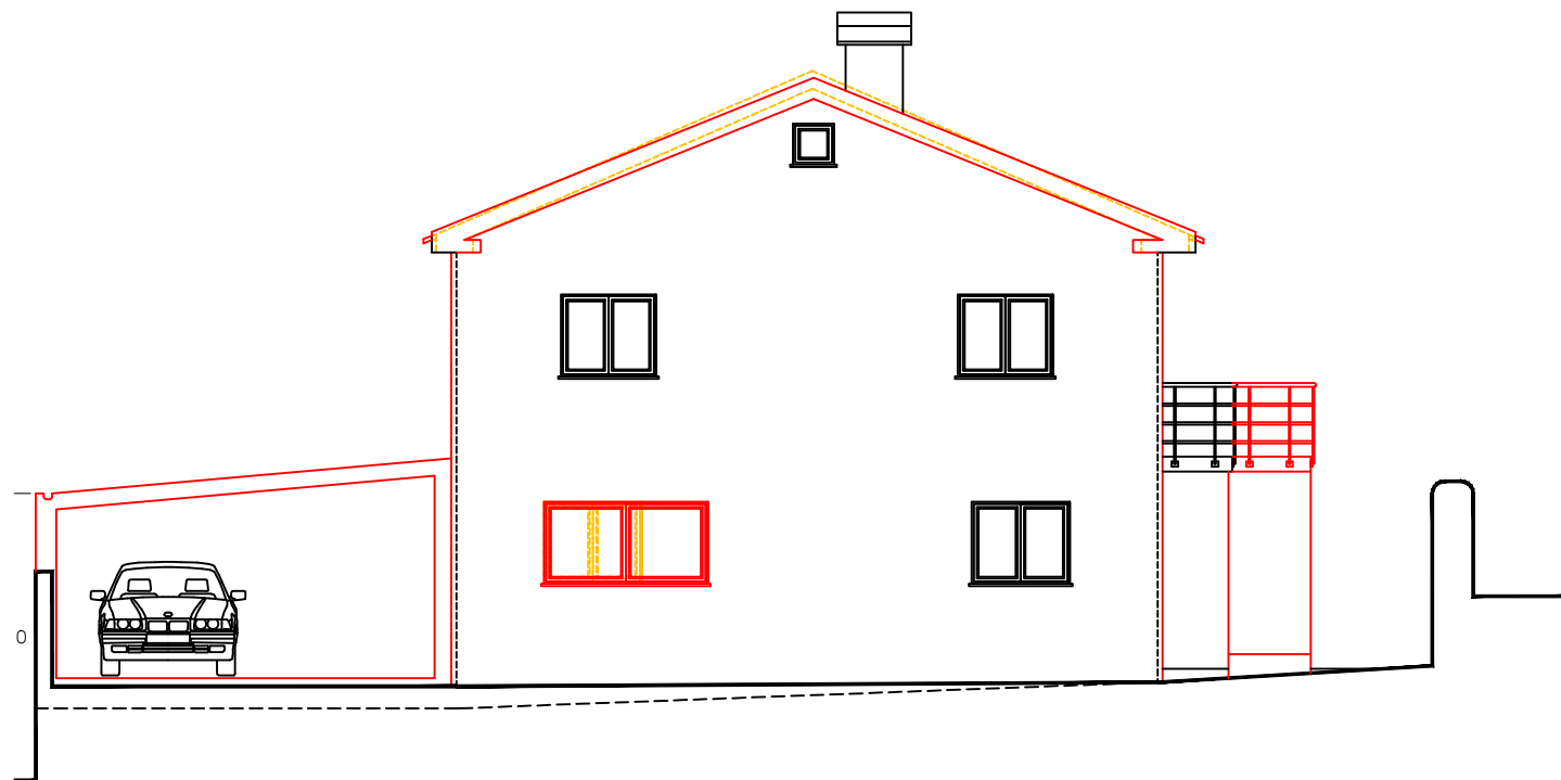
ALÇADO POENTE
