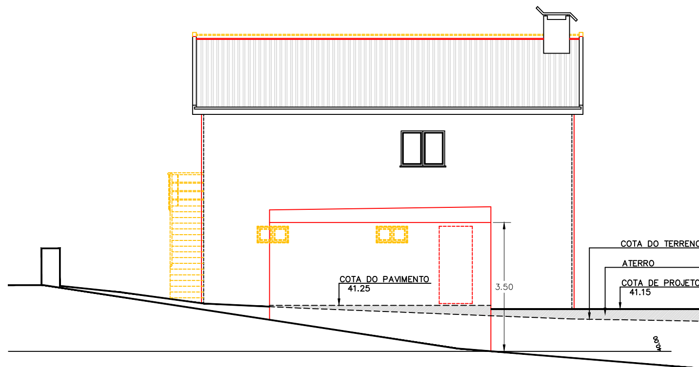
ALÇADO NORTE
