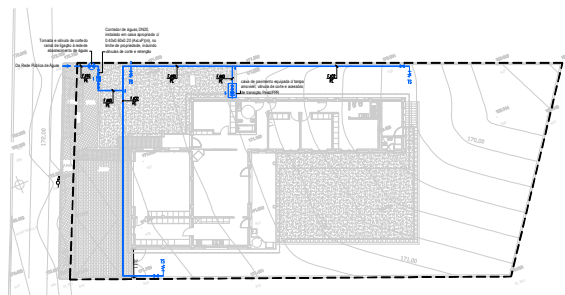
PLANTA DE IMPLANTAÇÃO mód. 100
