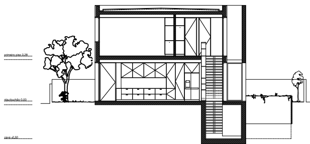
corte CC'
