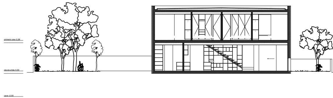
corte BB'
