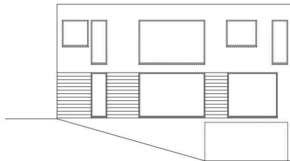
alçado nascente
