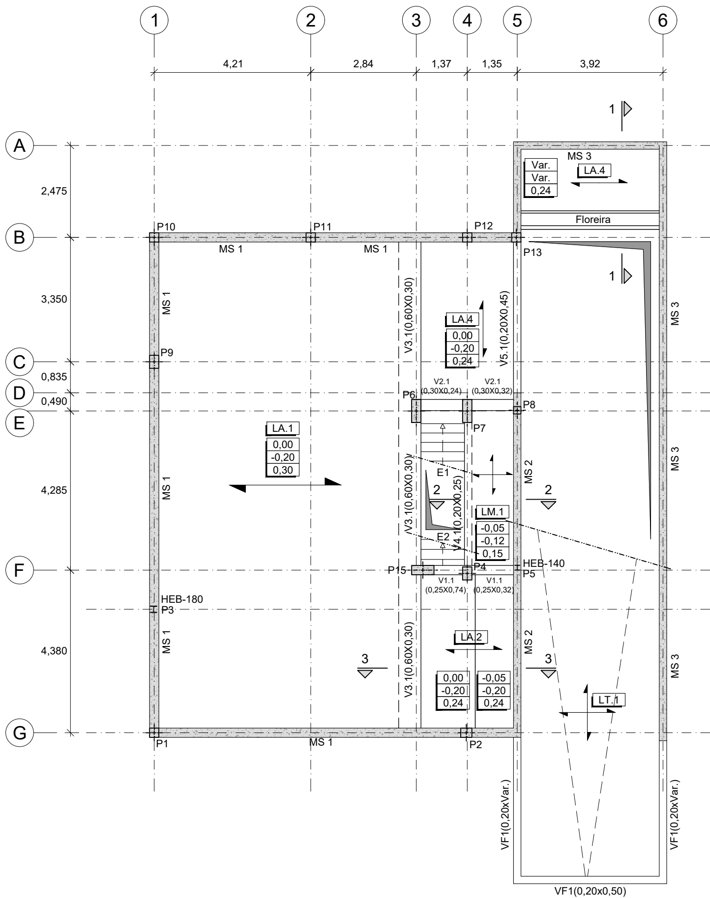
PLANTA ESTRUTURAL DO PISO 0 A1:1/100 ; A3:1/200
