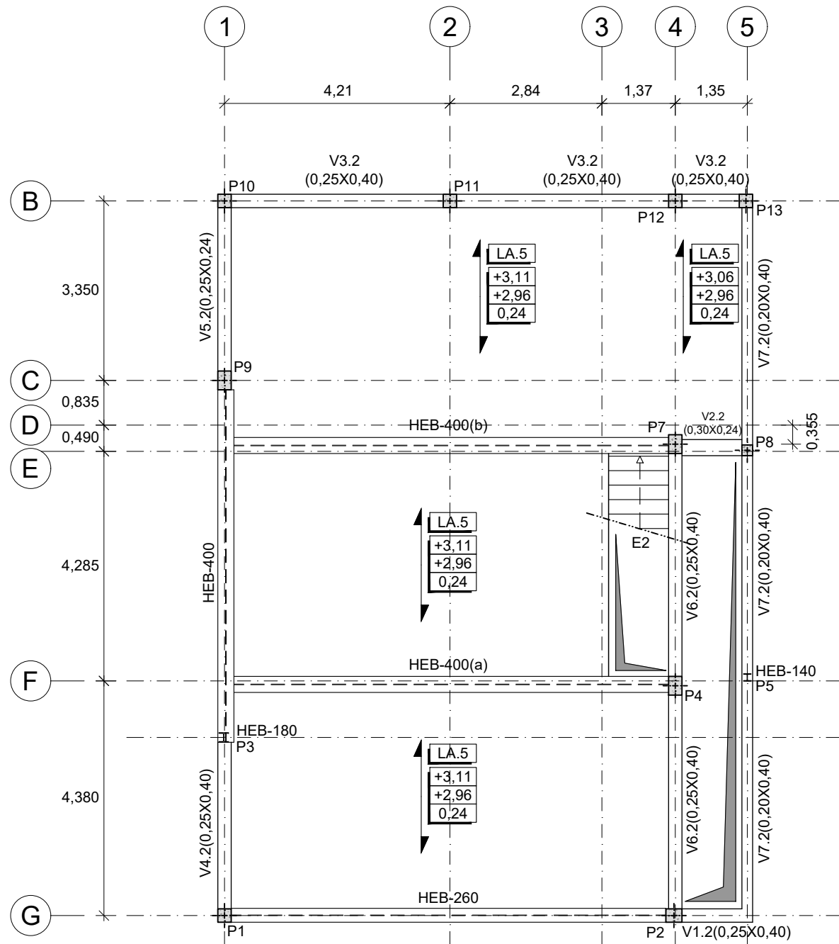
PLANTA ESTRUTURAL DO PISO 1 A1:1/100 ; A3:1/200
