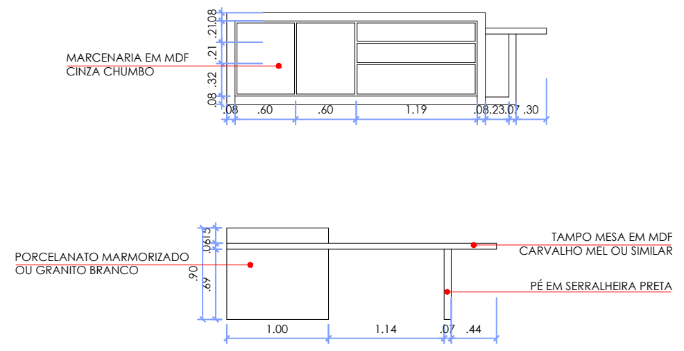
DETALHES ILHA E MESA DE JANTAR ESCALA 1:50
