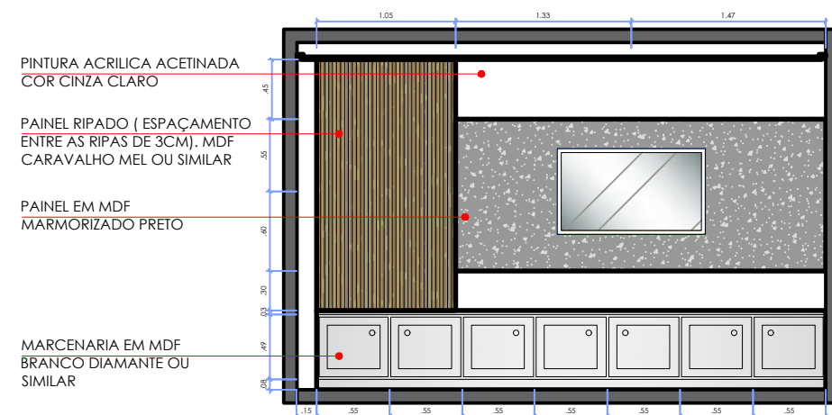
ELEVAÇÃO A - QUARTO SUÍTE ESCALA 1:50
