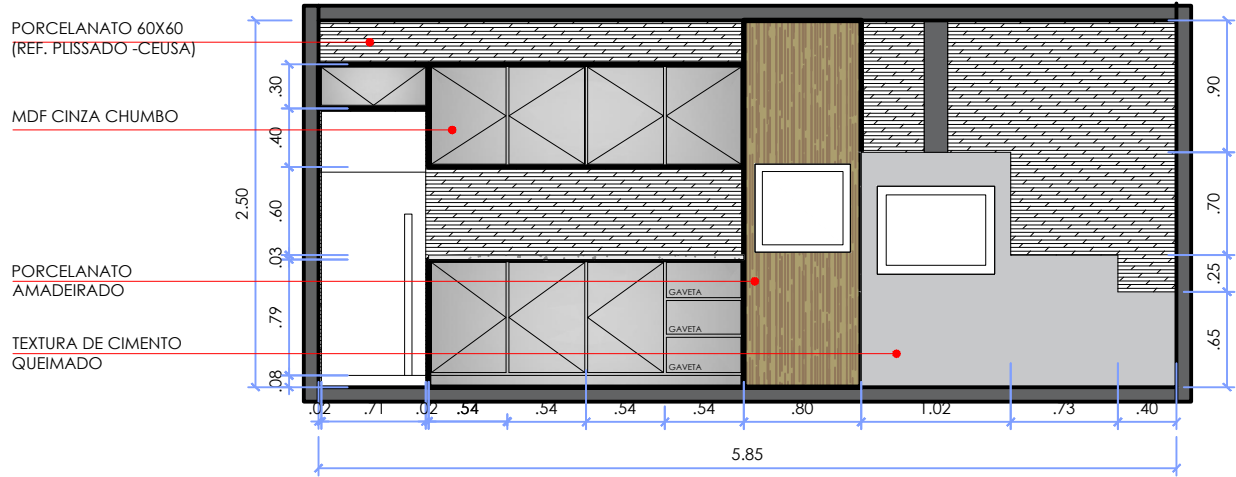
ELEVAÇÃO - ÁREA GOURMET ESCALA 1:50
