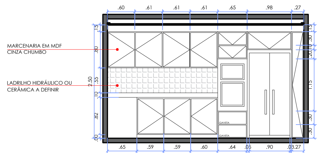
ELEVAÇÃO B - COZINHA ESCALA 1:50
