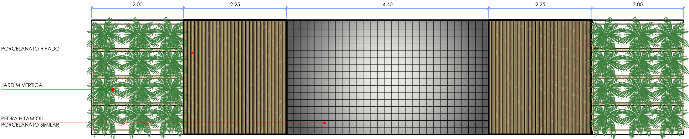
ELEVAÇÃO - ÁREA EXTERNA (MURO PISCINA) ESCALA 1:50
