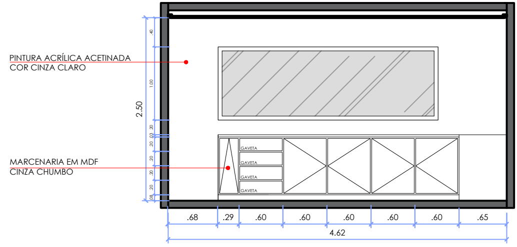
ELEVAÇÃO A - COZINHA ESCALA 1:50
