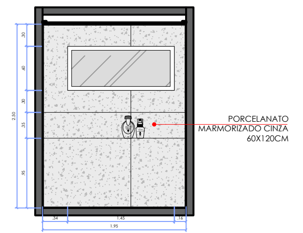
ELEVAÇÃO C - BANHO ESCALA 1:50
