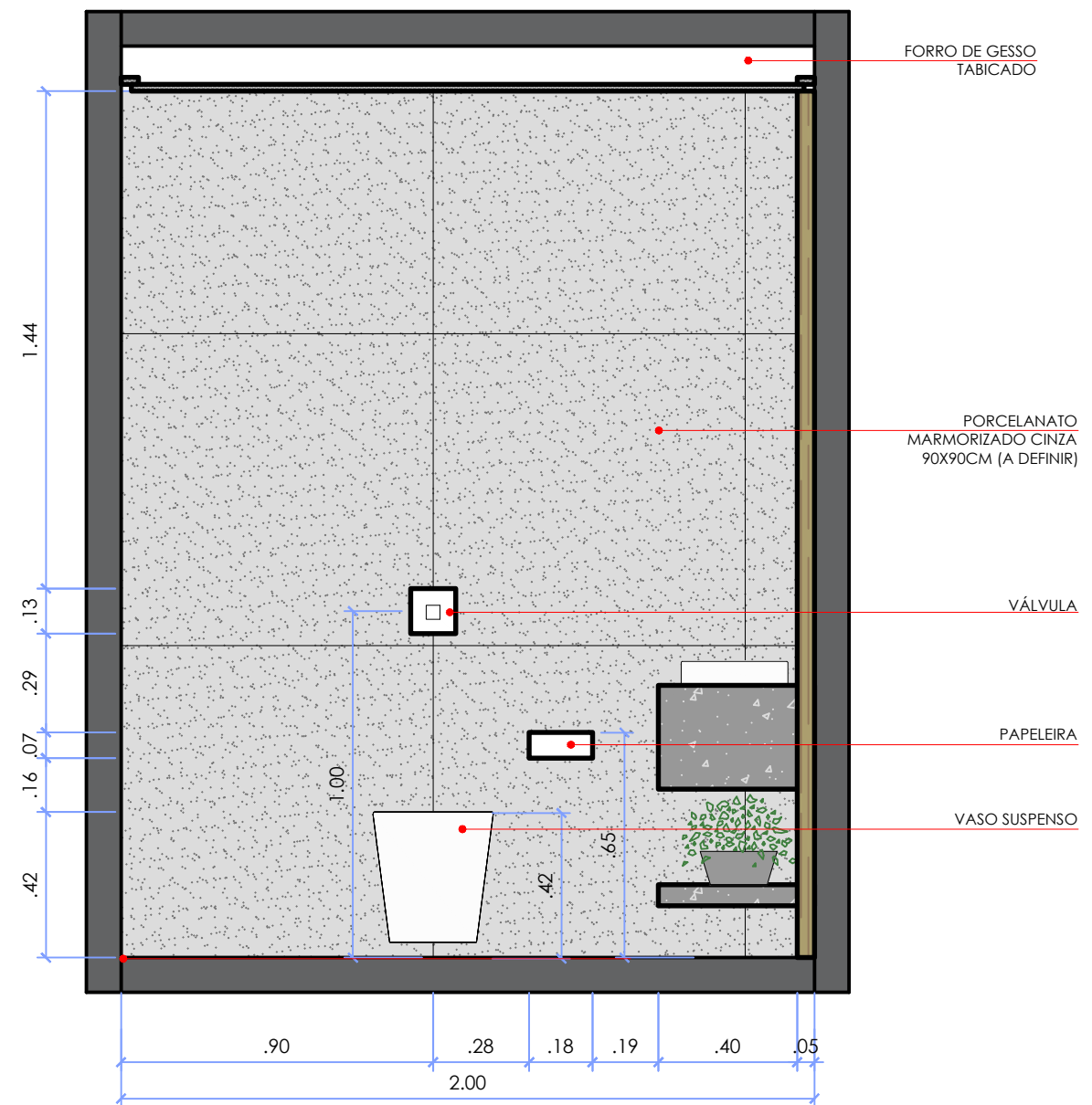
ELEVAÇÃO B - LAVABO ESCALA 1:20
