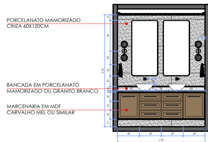
ELEVAÇÃO A - BANHO ESCALA 1:50
