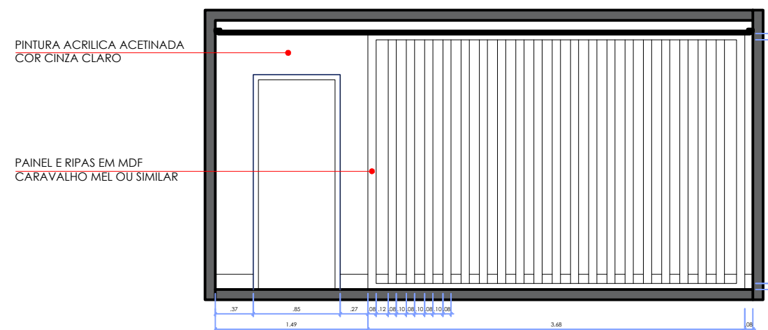
ELEVAÇÃO B - QUARTO SUÍTE ESCALA 1:50
