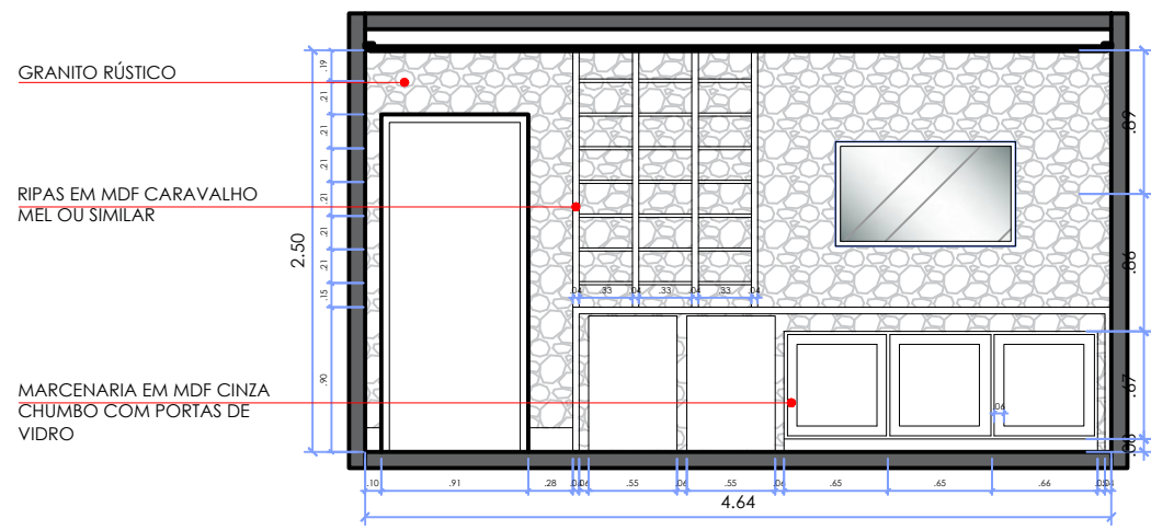
ELEVAÇÃO C - COZINHA ESCALA 1:50
