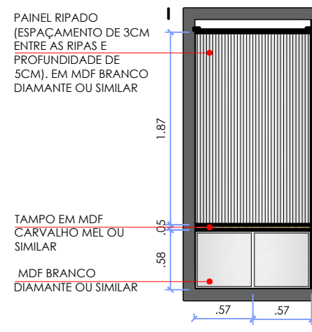
ELEVAÇÃO HALL ESCALA 1:50
