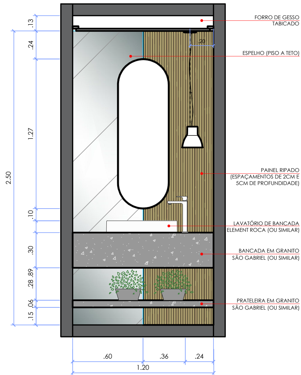
ELEVAÇÃO A - LAVABO ESCALA 1:20
