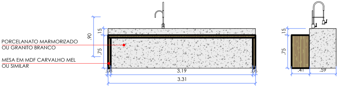
ELEVAÇÃO BANCADA - ÁREA GOURMET ESCALA 1:50
