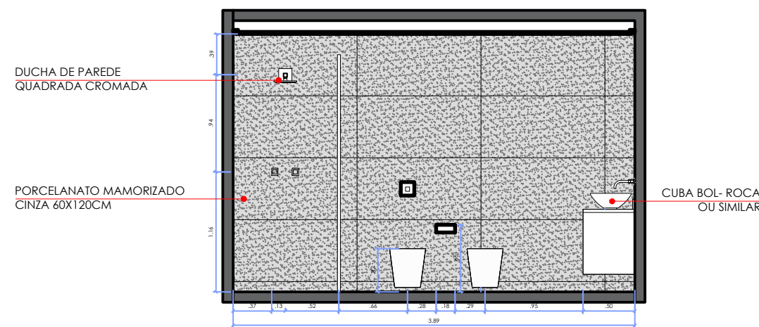
ELEVAÇÃO B- BANHO ESCALA 1:50
