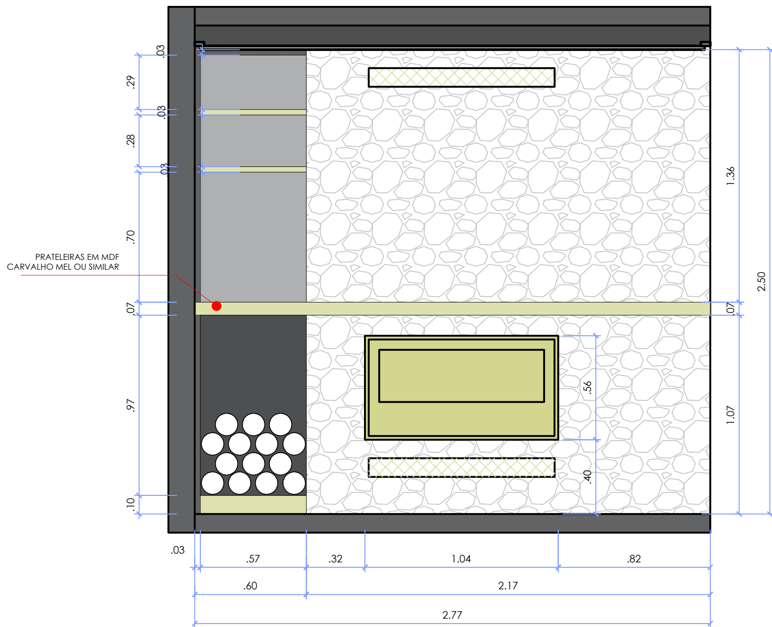
VISTA FRONTAL - LAREIRA ESCALA 1:20
