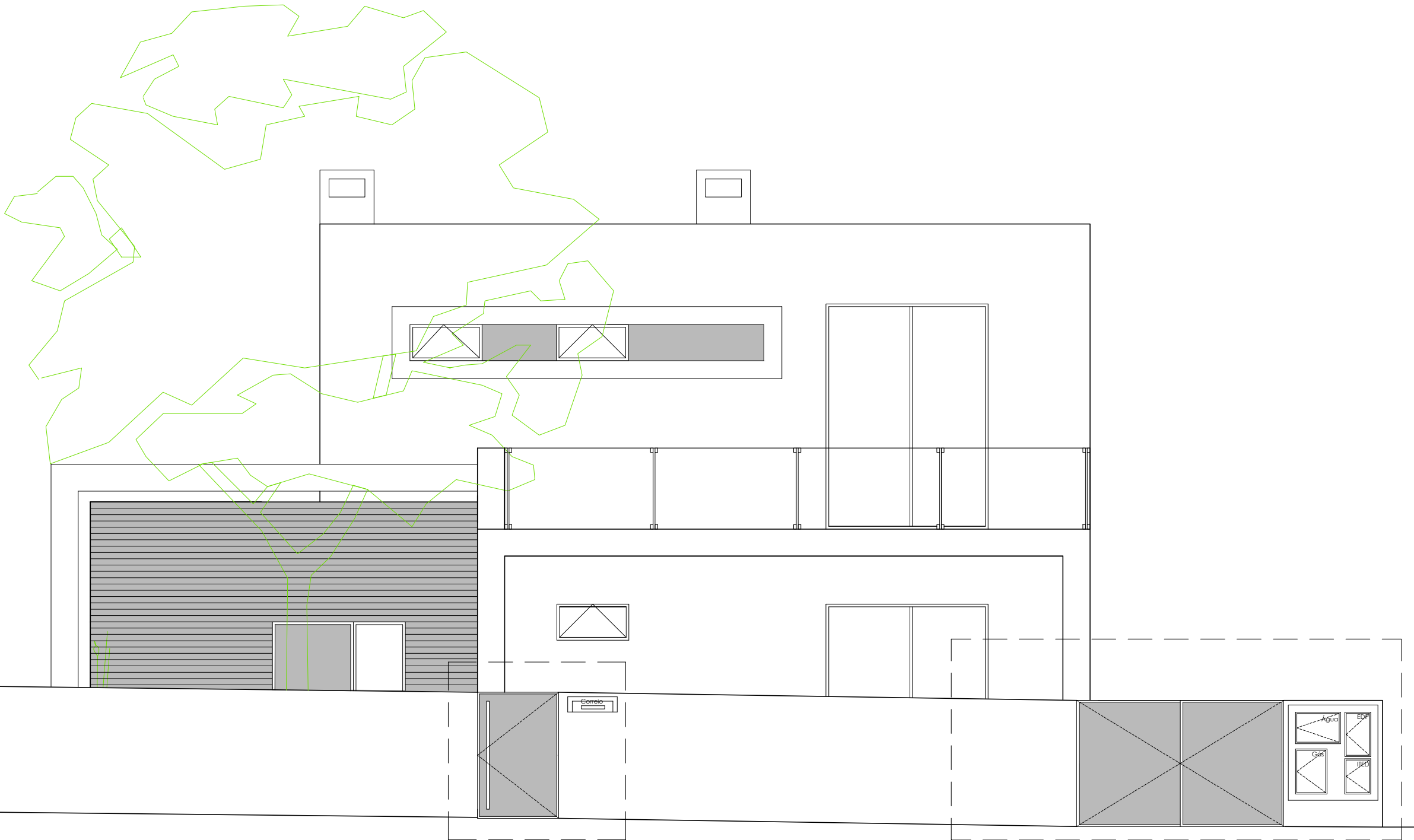
Alçado Principal
