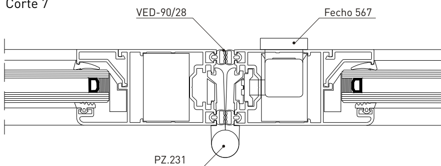
Corte 7
