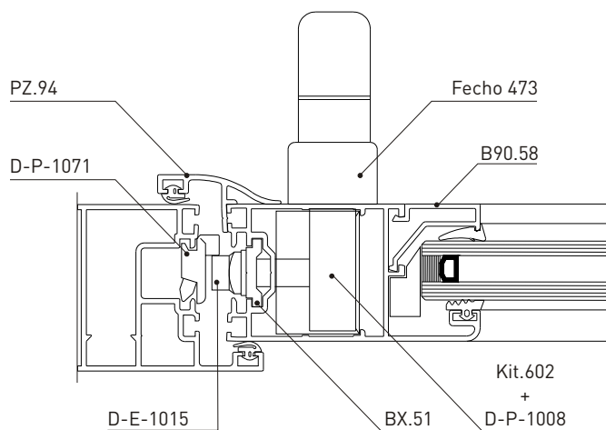
Corte 6a
