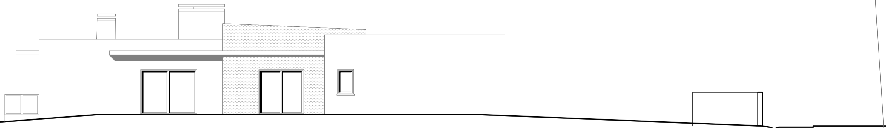
ALÇADO SW
