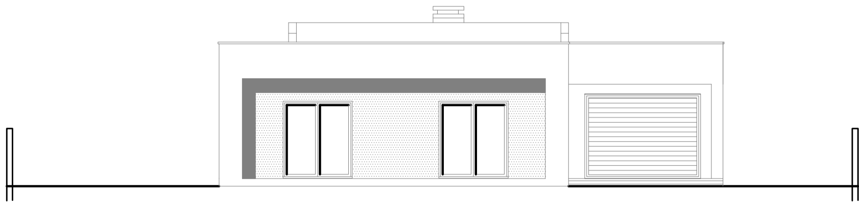
ALÇADO FRENTE ESTRADA
