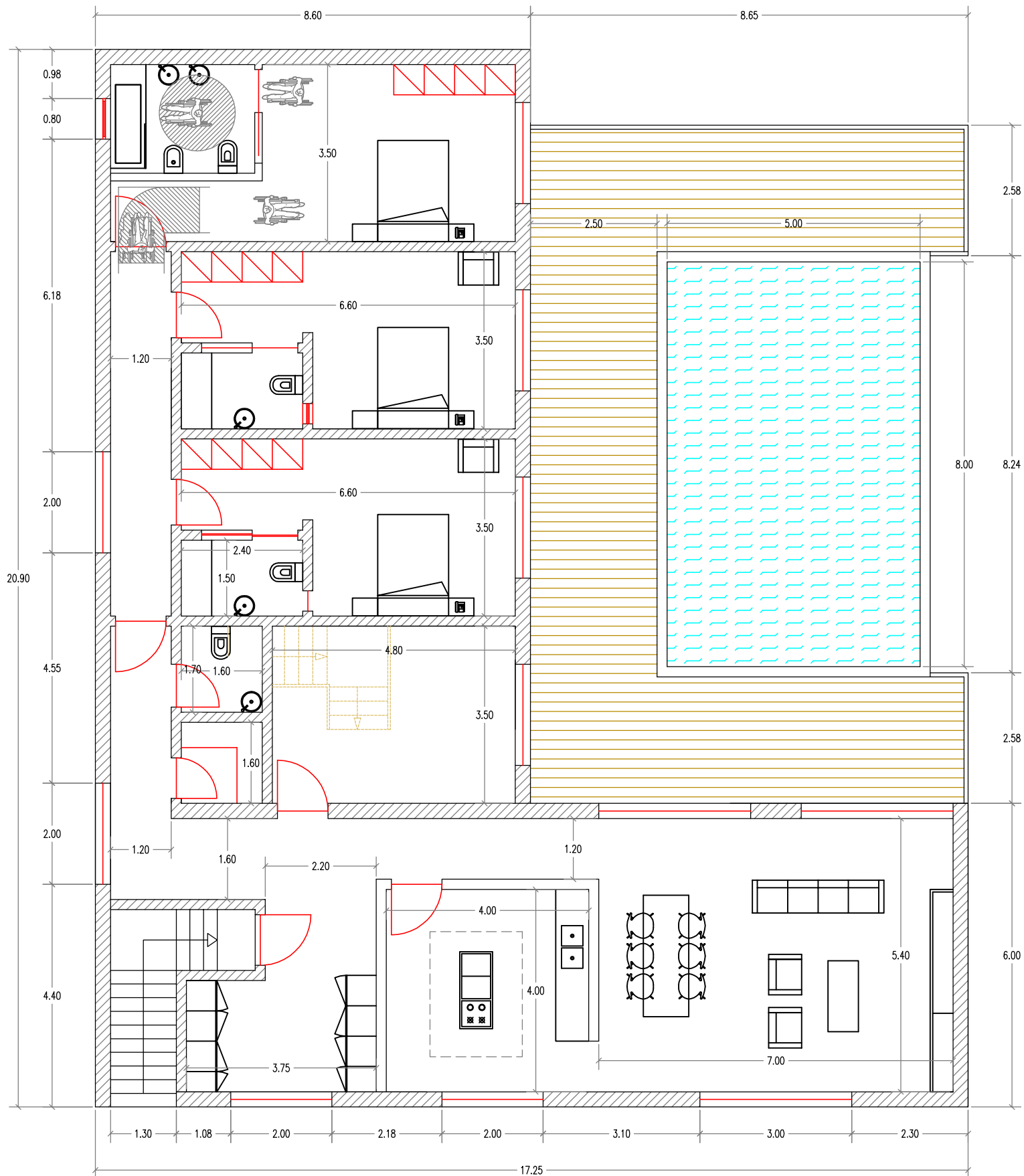
PLANTA DO ANDAR
