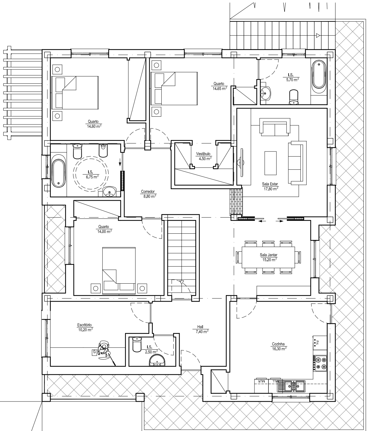
PLANTA DO R/CHÃO
