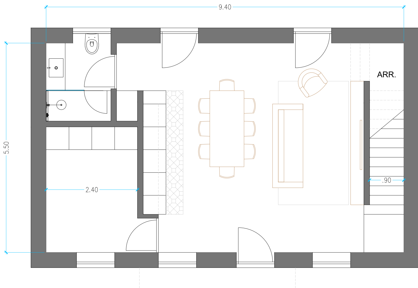
PLANTA DO 1ºANDAR
