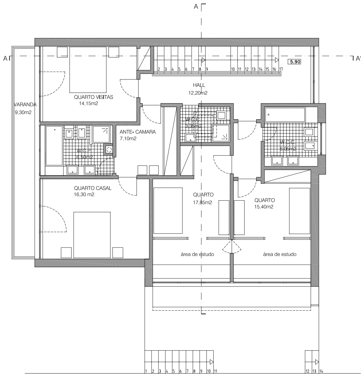
PLANTA PISO 2
