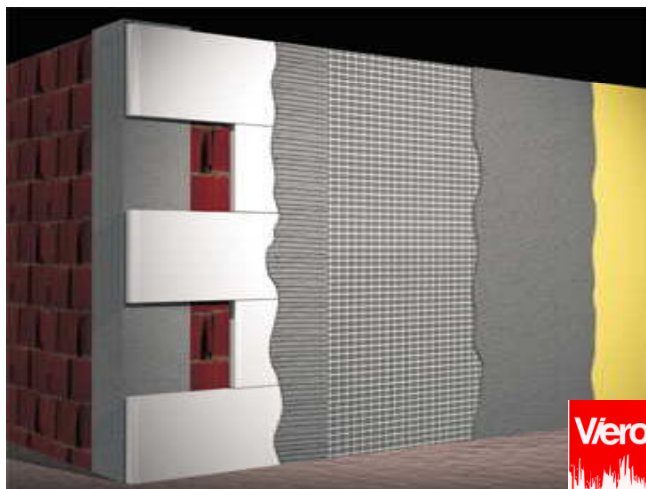
CORTE DO SISTEMA DE ISOLAMENTO TÉRMICO PELO EXTERIOR "CAPPOTTO" - VIERO
