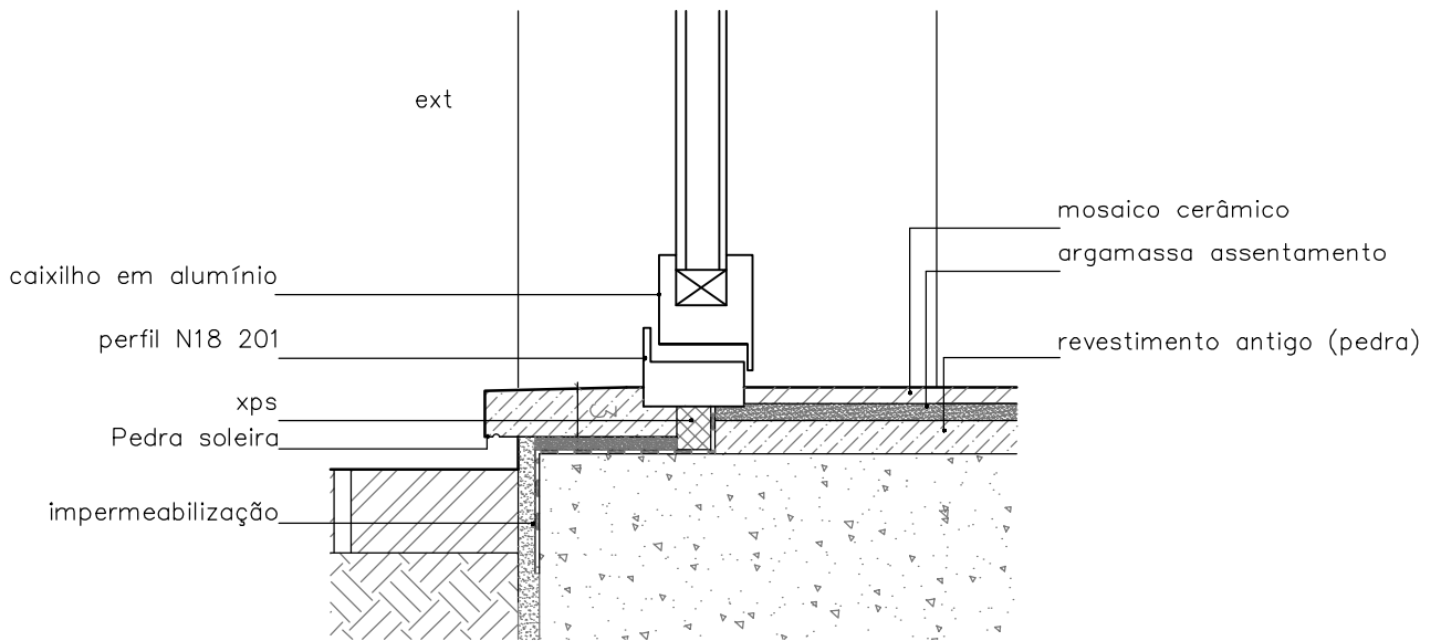
Pormenor soleira Janela sacada
