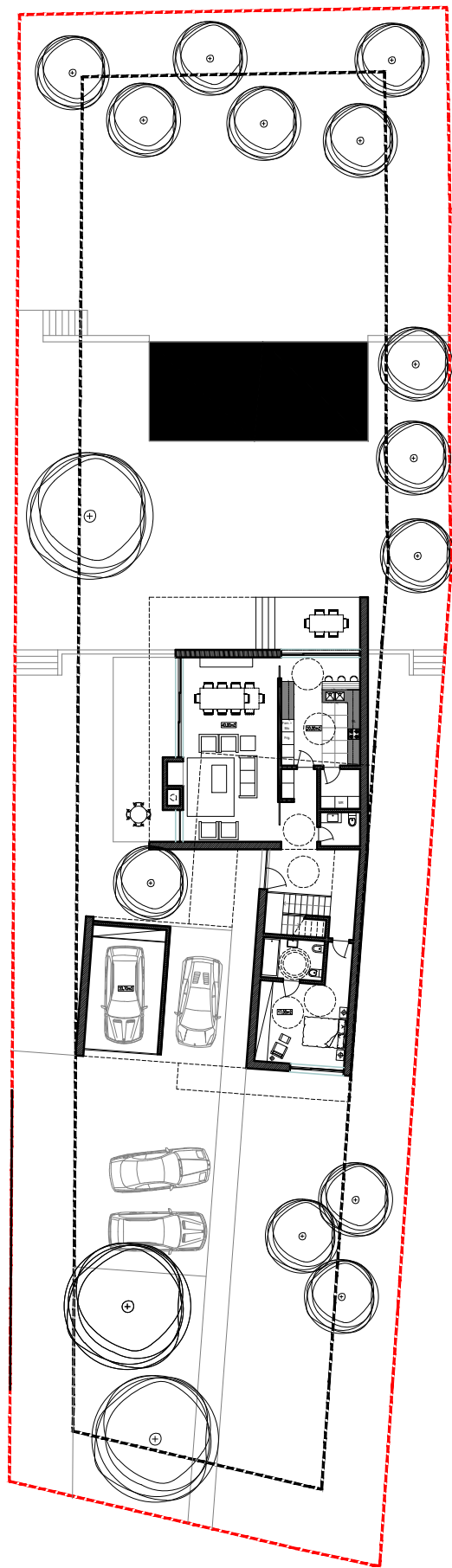
PLANTA R/CH ÁB Const. — 142m 2 +25m 2
