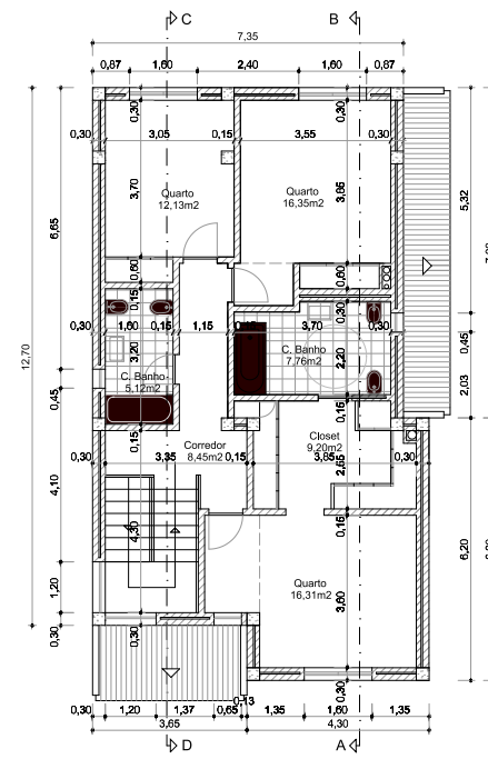
PLANTA DO 1º ANDAR
