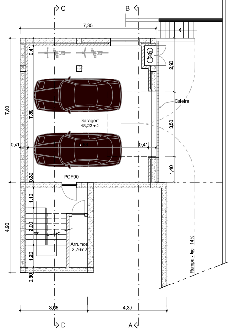
PLANTA DA CAVE
