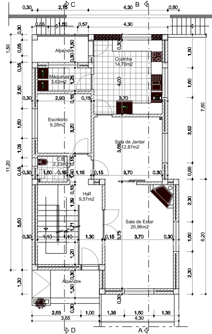
PLANTA DO R/CHÃO
