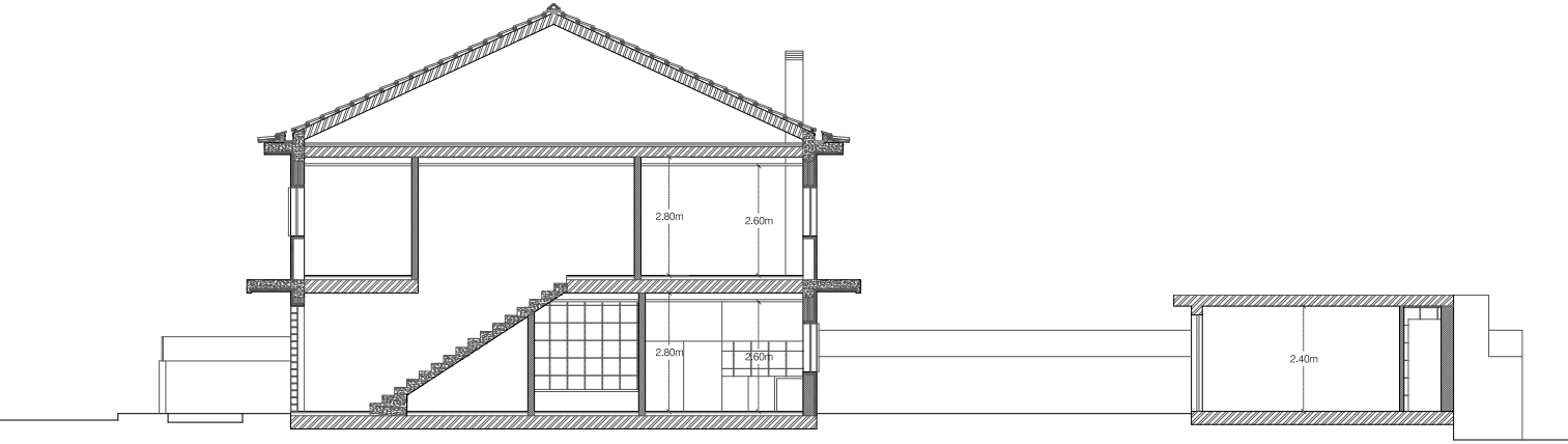
CORTE A-B
