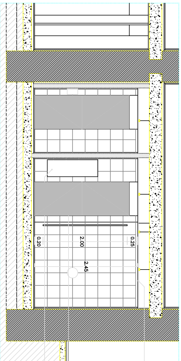
CORTE 4
