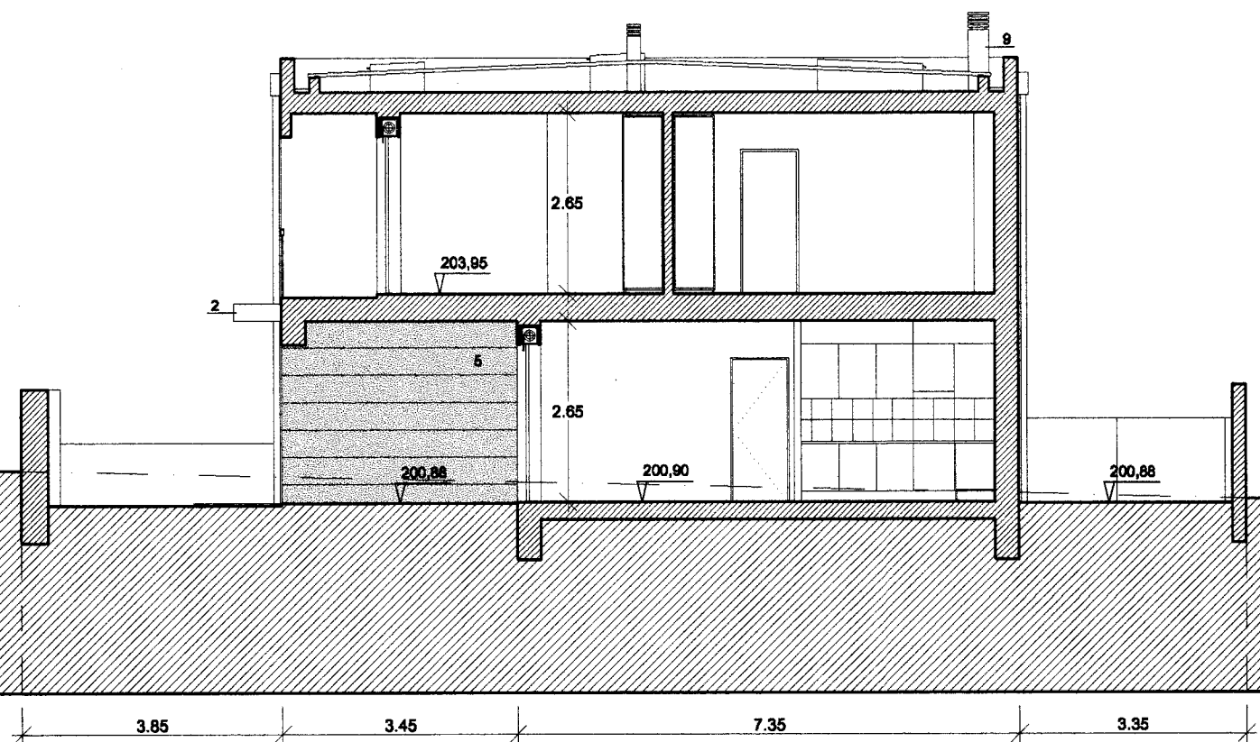
Corte C2
