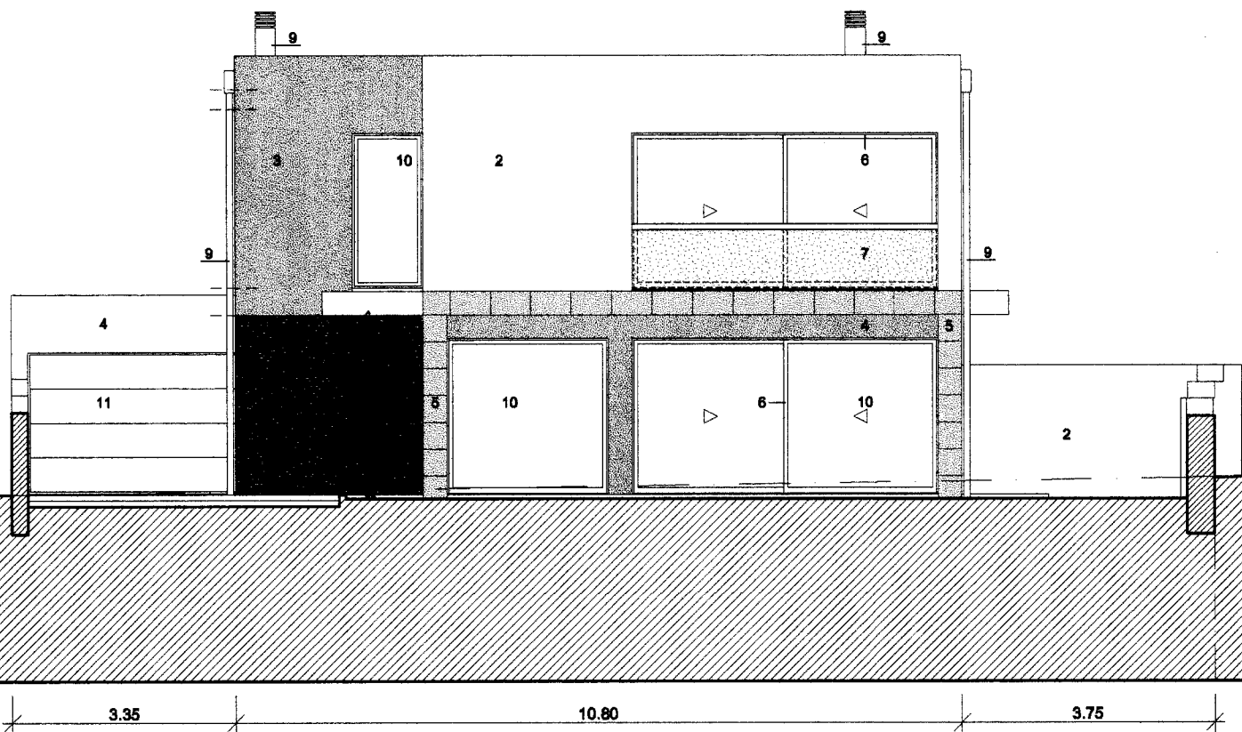
Corte C1
