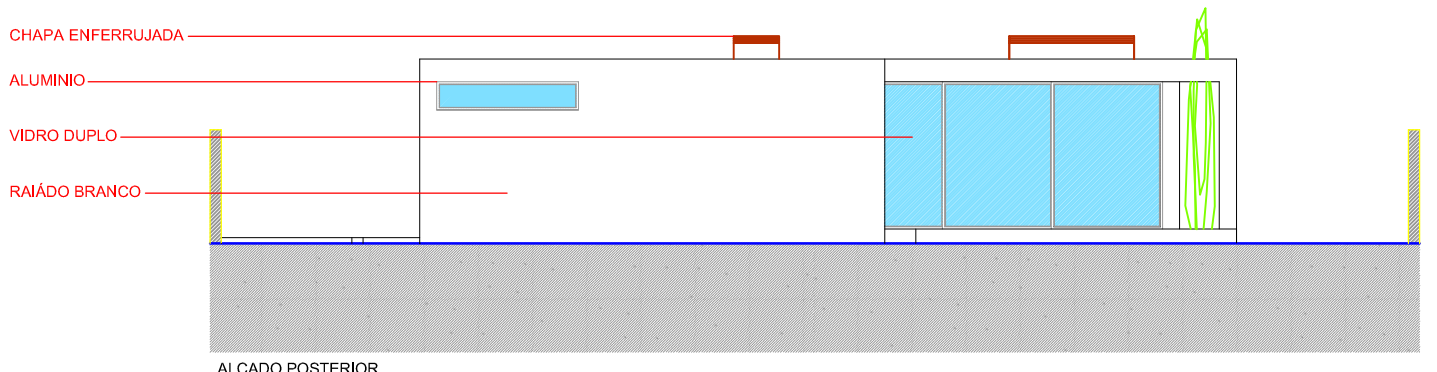
ALÇADO POSTERIOR
