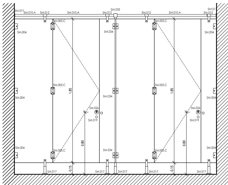
ALÇADO
