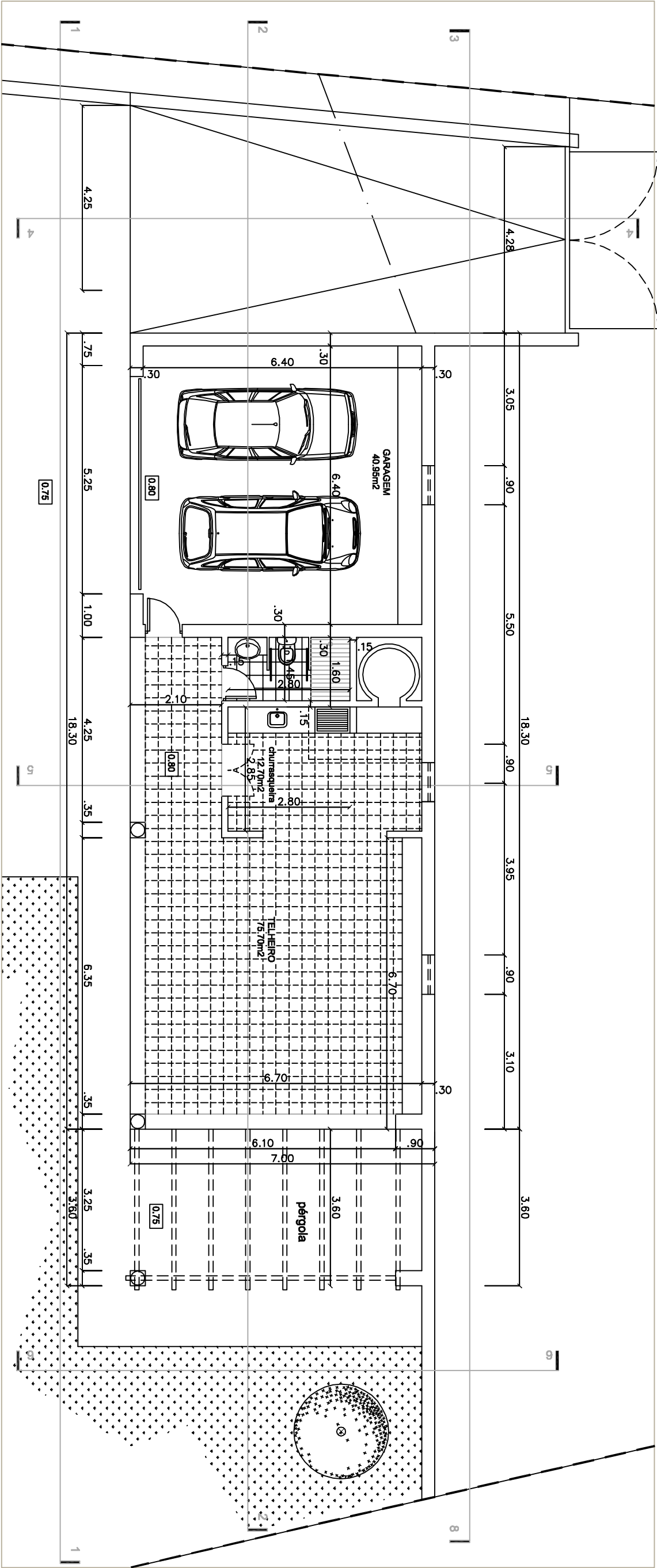
PLANTA TERREA
