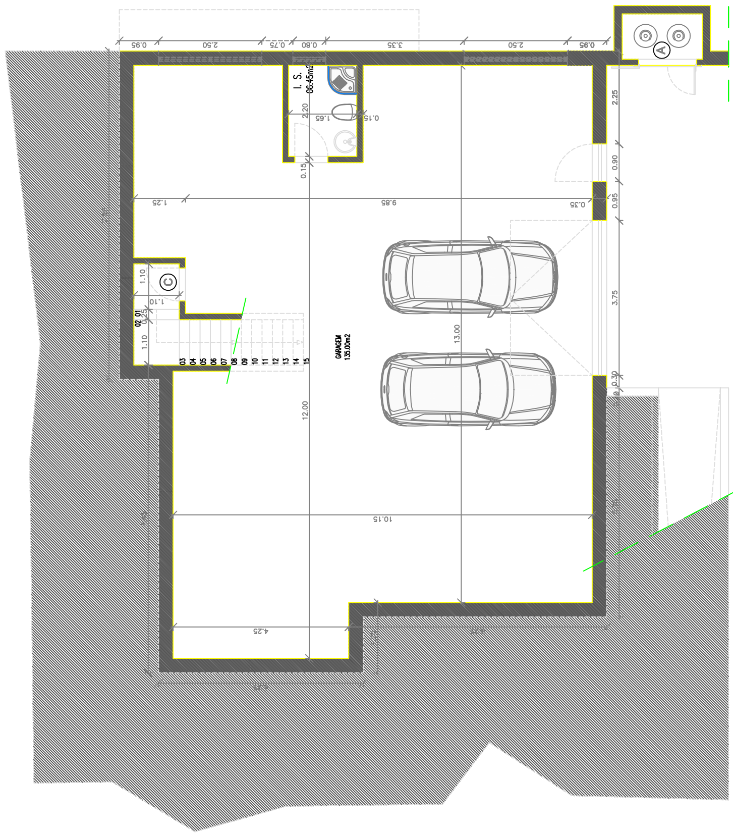
PLANTA DA CAVE
