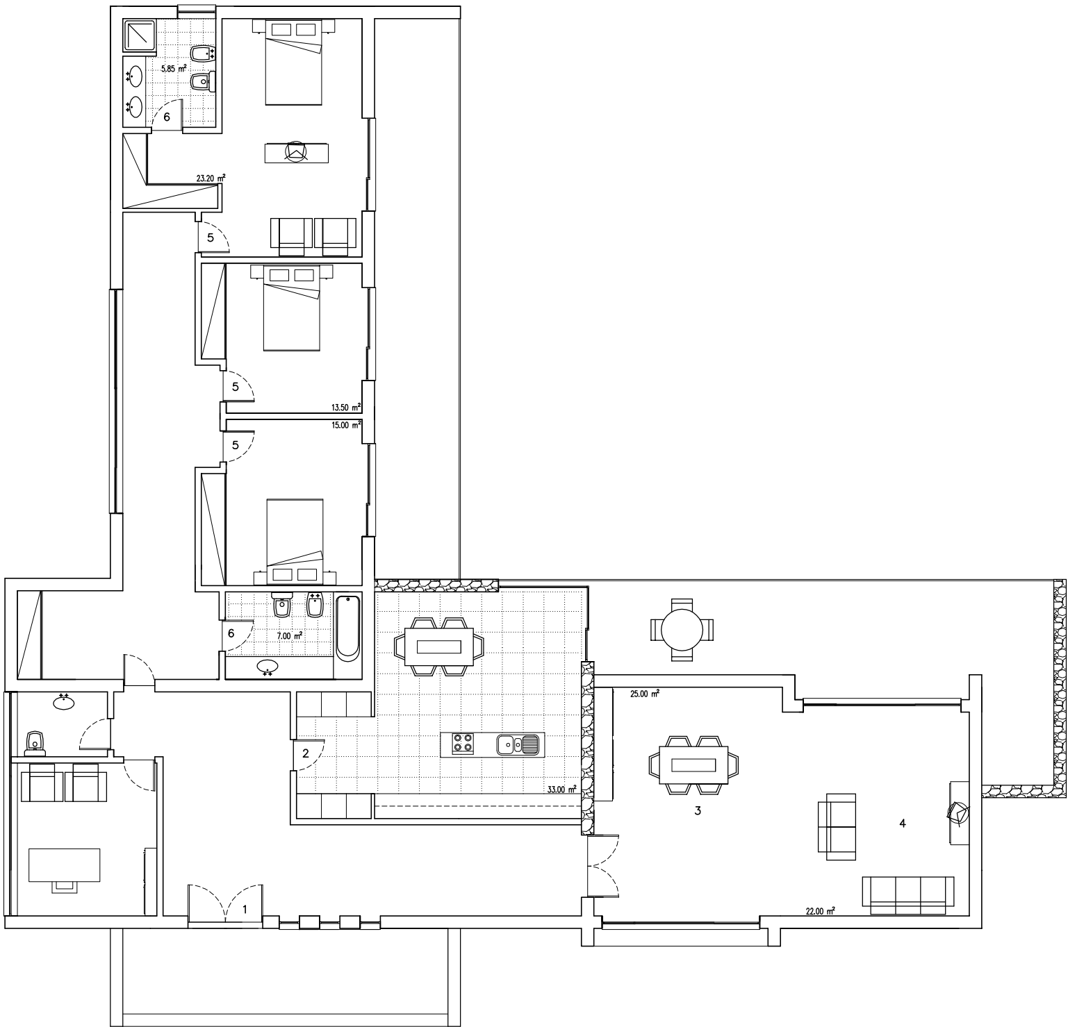
PLANTA DO RÉS-DO-CHÃO
