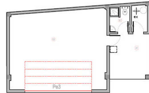
PLANTA (ANEXO)
