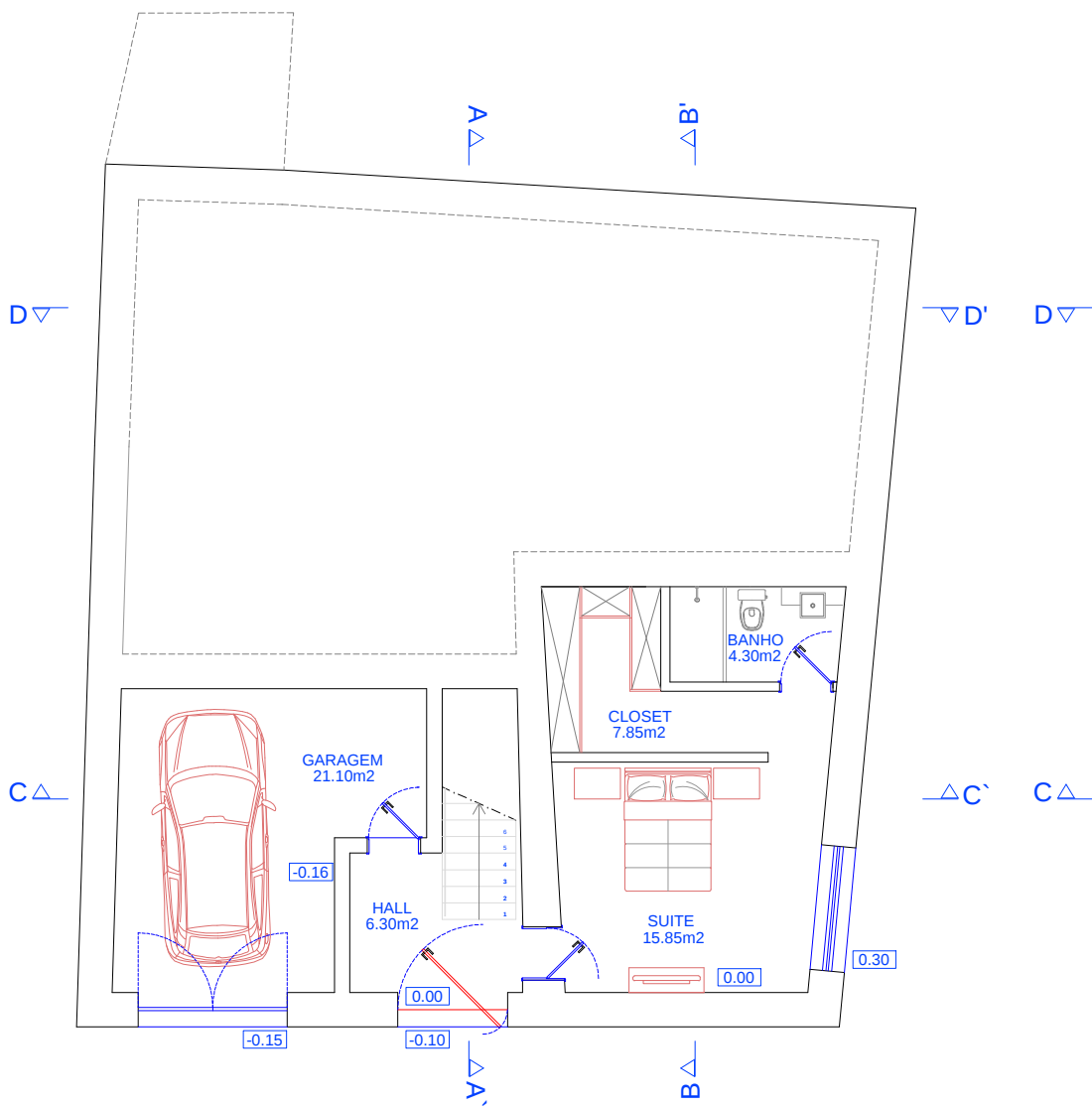
Planta R° s-do-Chão esc.100
