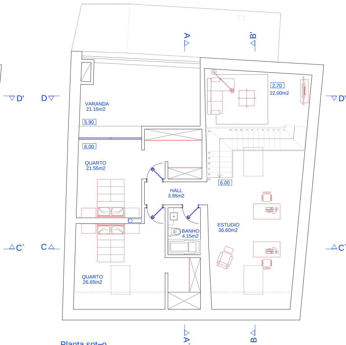
Planta sótão esc.100
