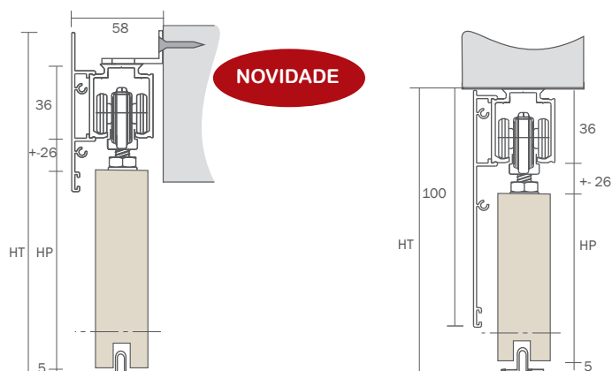
Fixação à parede
