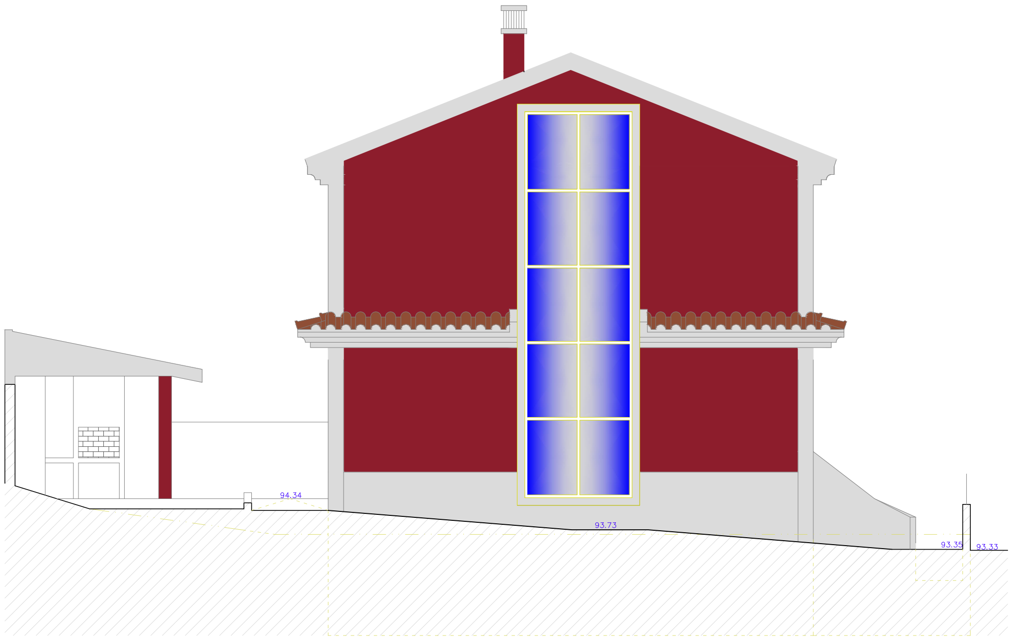
Alçado Lateral Esquerdo
