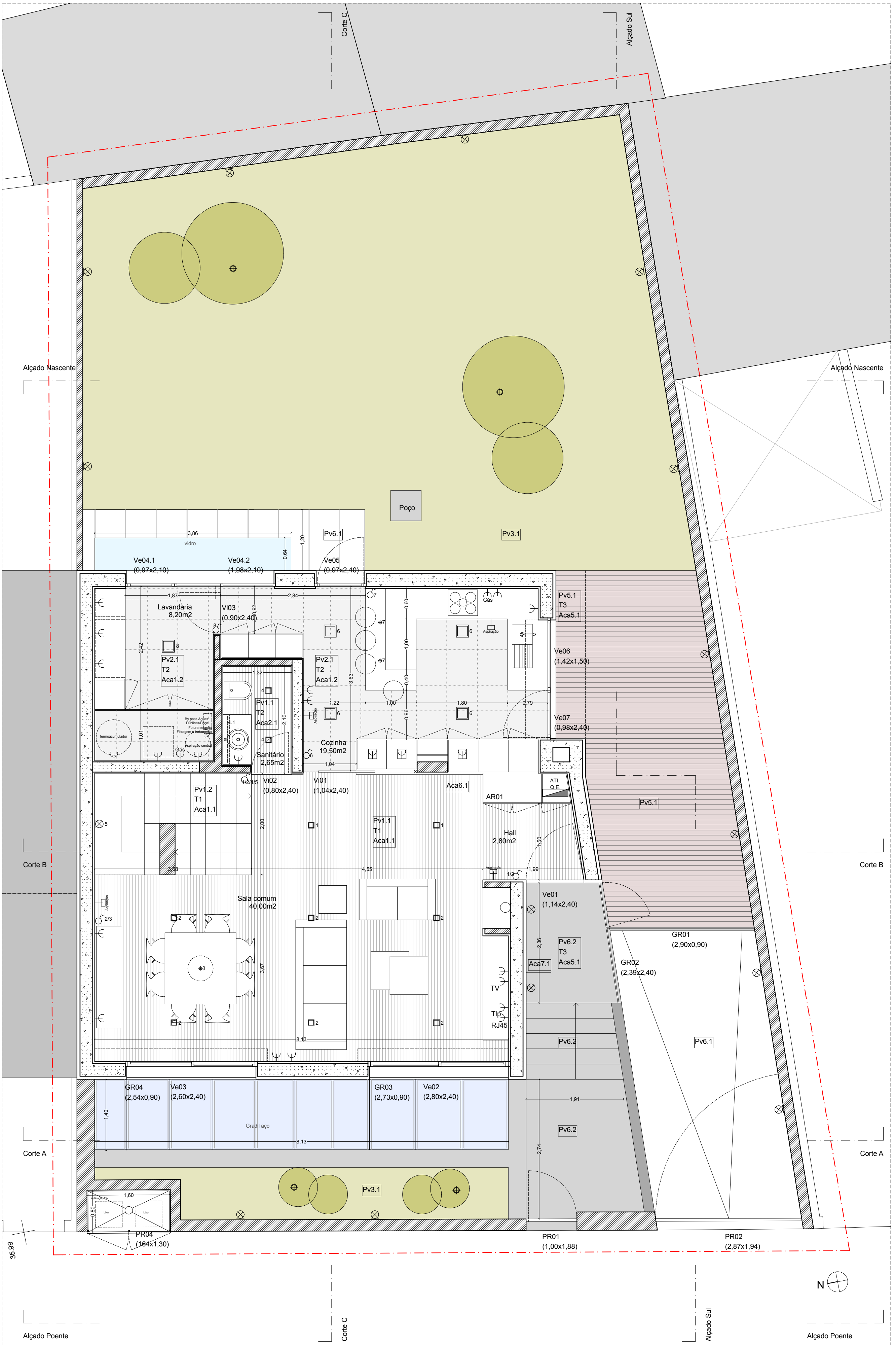
Planta Piso 0 1:50
