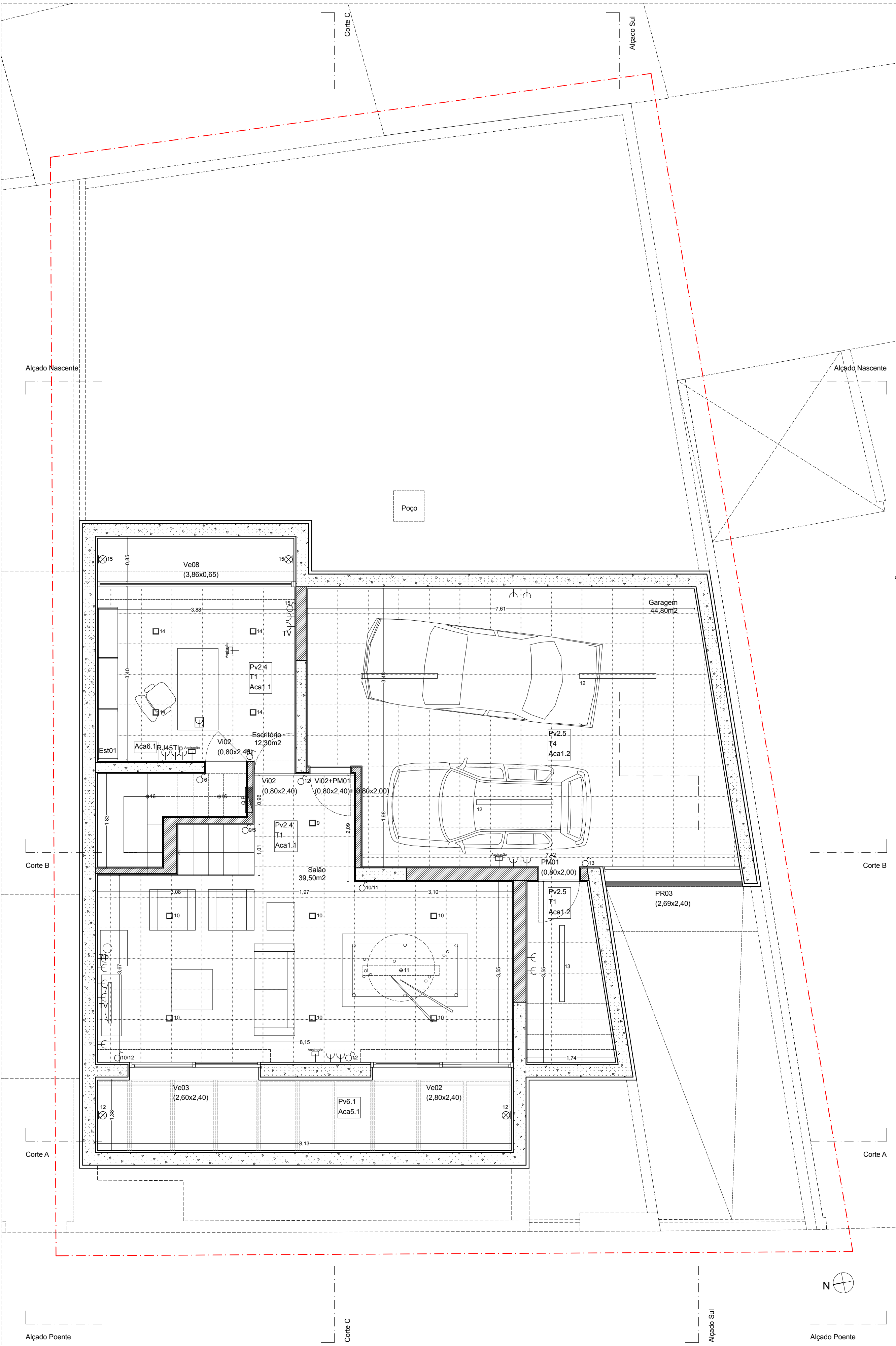
Planta Piso -1 1:50
