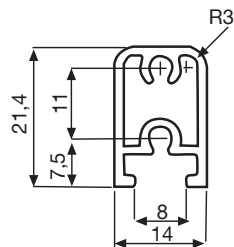
Perfil soporte de estantes / Shelves support profile
