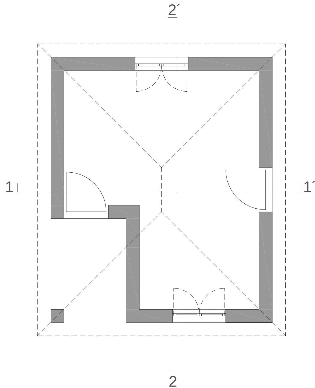
PLANTA TERREA
