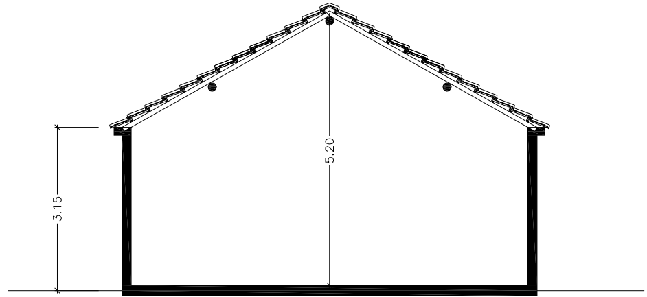
corte
