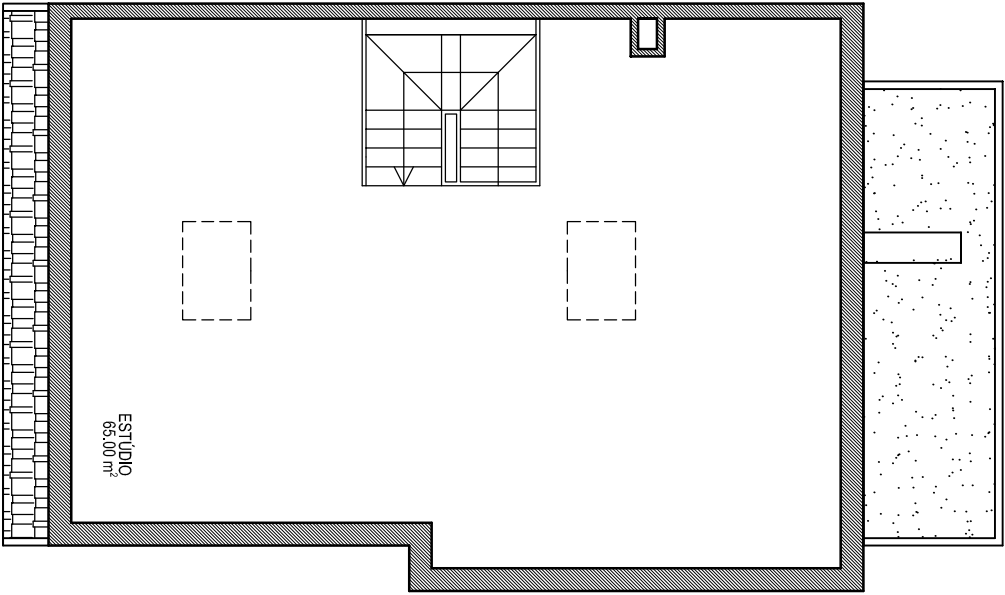
PLANTA DO SOTÃO
