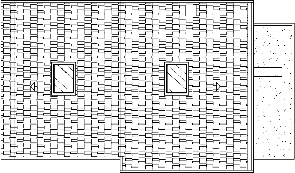
PLANTA DA COBERTURA
