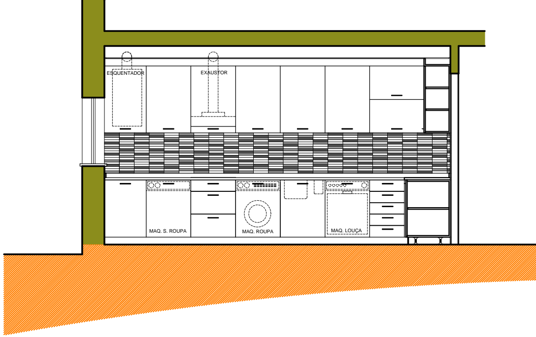
VISTA 1 - ESC 1/50
