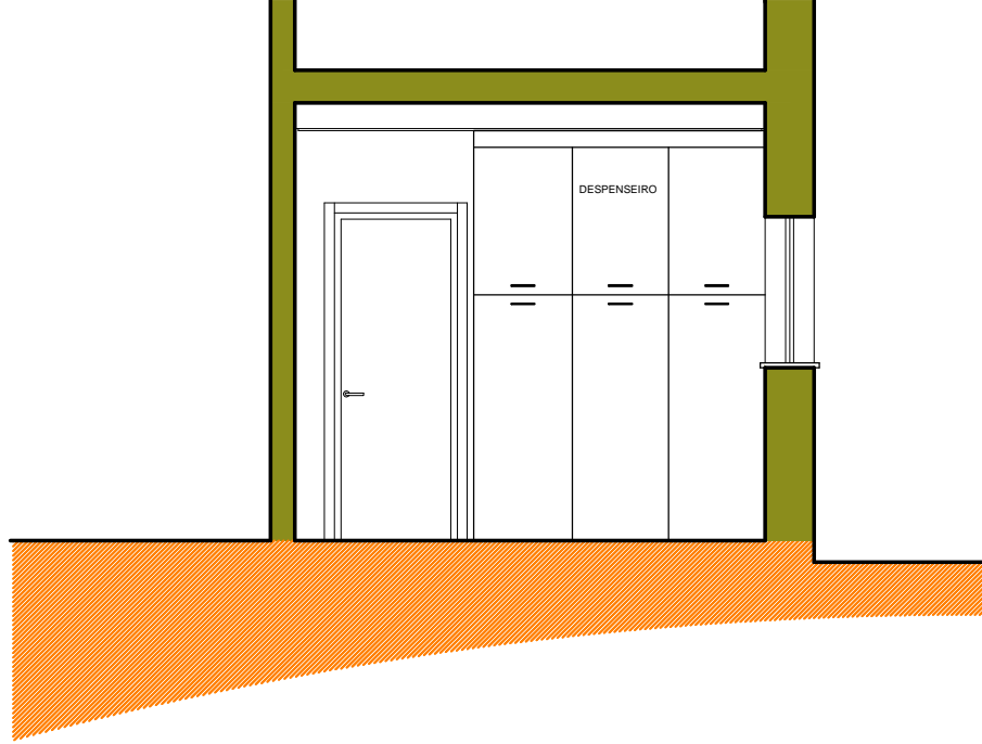
VISTA 3 - ESC 1/50
